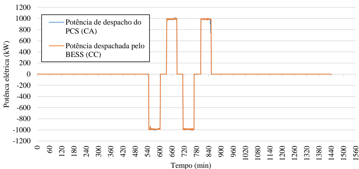
Figura 5 - Teste de capacidade para 1C.
