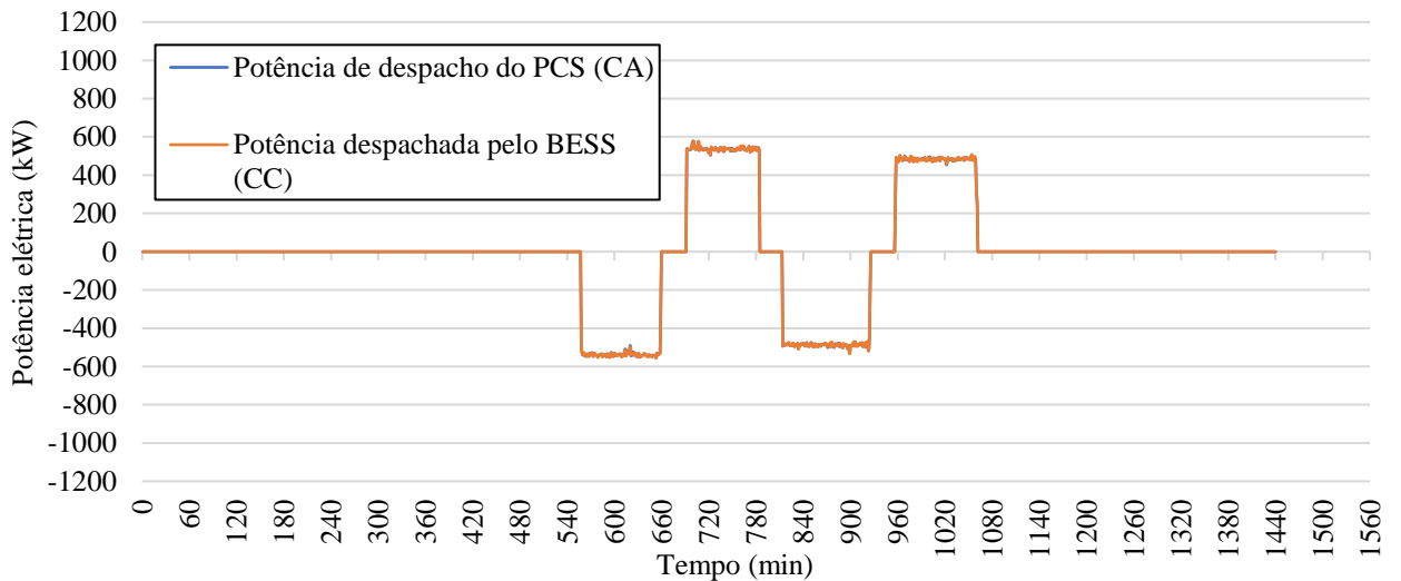
Figura 4 - Teste de capacidade para \frac{1}{2}C .
