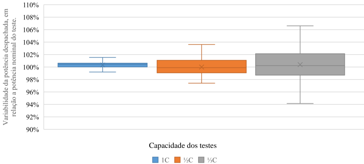
Figura 6 - Variabilidade da potência despachada no sistema durante os testes de capacidade para diferentes despachos.
