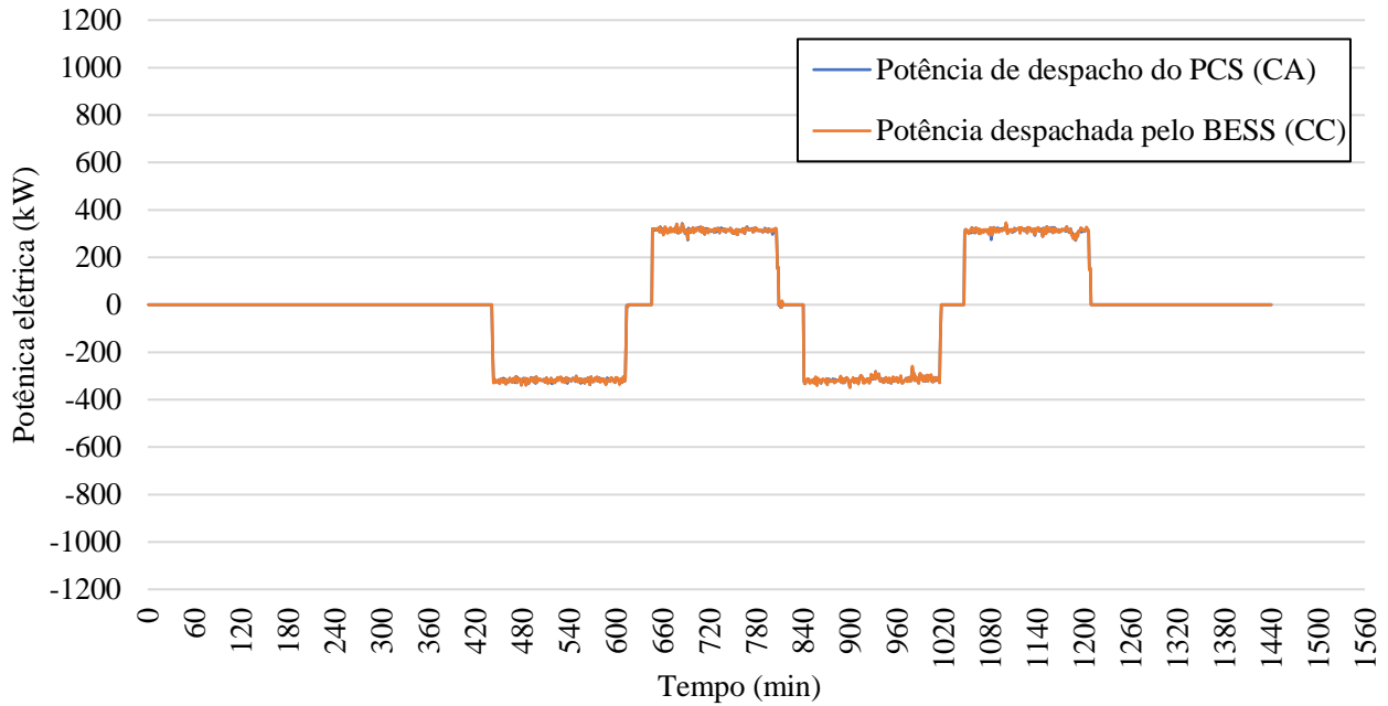
Figura 3 - Teste de capacidade para \frac{1}{3}C .
