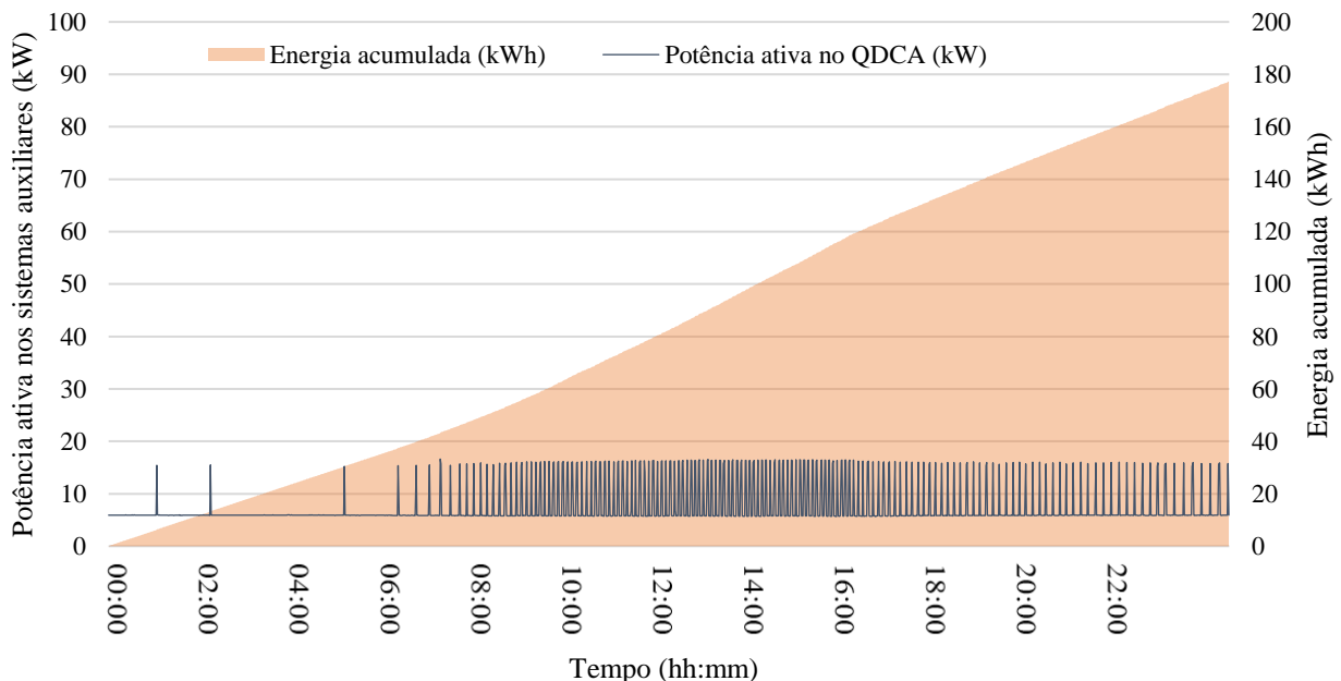
Figura 7 - Demanda e consumo energético dos sistemas auxiliares do BESS ao longo de um dia sem operação de despacho de bateria.
