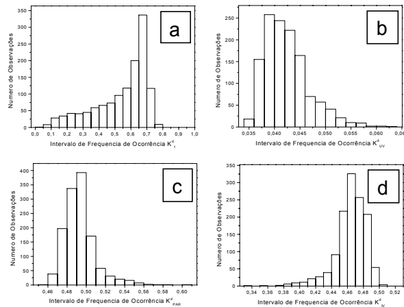
Figura 3 - Histograma de frequência das frações diárias: (a) K_T^d ; (b) K_{UV}^d ; (c) K_{PAR}^d e (d) K_{IV}^d .
