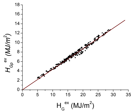
Figura 2 - Correlação da radiação H_{Gp}^{ex} em função de H_G^{ex} .
