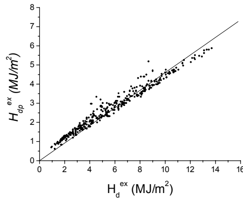
Figura 4 - Correlação da radiação H_{dp}^{ex} em função de H_d^{ex} .
