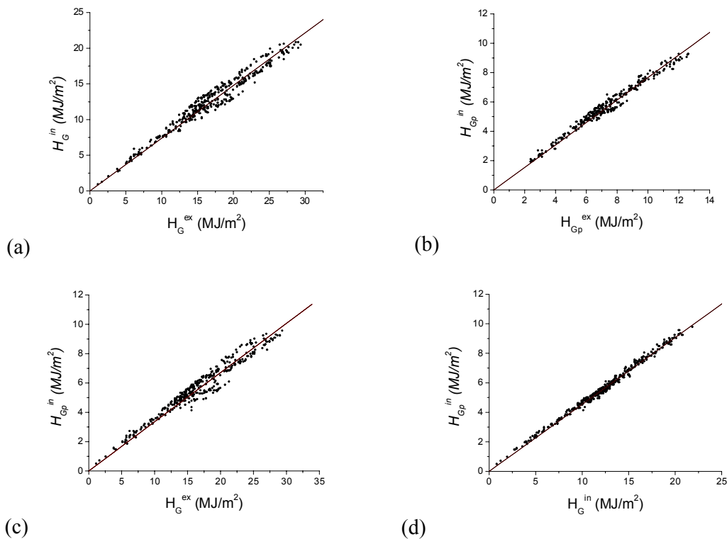
Figura 1 - Correlações das radiações H_G^{in} e H_{Gp}^{in} em função de H_{Gp}^{ex} , H_G^{ex} e H_G^{in} .
