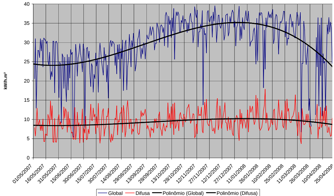
Fig.5 – Comparação entre as somas diárias das radiações global e difusa em Natal-RN entre 01/05/2007 e 25/04/2008.
