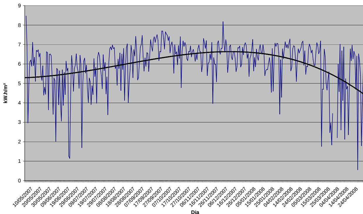
Fig.3 – Irradiação solar em Natal-RN entre 01/05/2007 e 25/04/2008.
