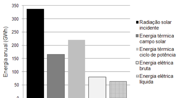
Figura 4 - Energia em base anual para planta com aquecimento auxiliar
