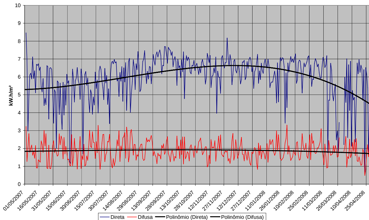
Fig.15 – Comparação entre médias global e difusa da irradiação solar global em Natal-RN entre 01/05/2007 e 25/04/2008.
