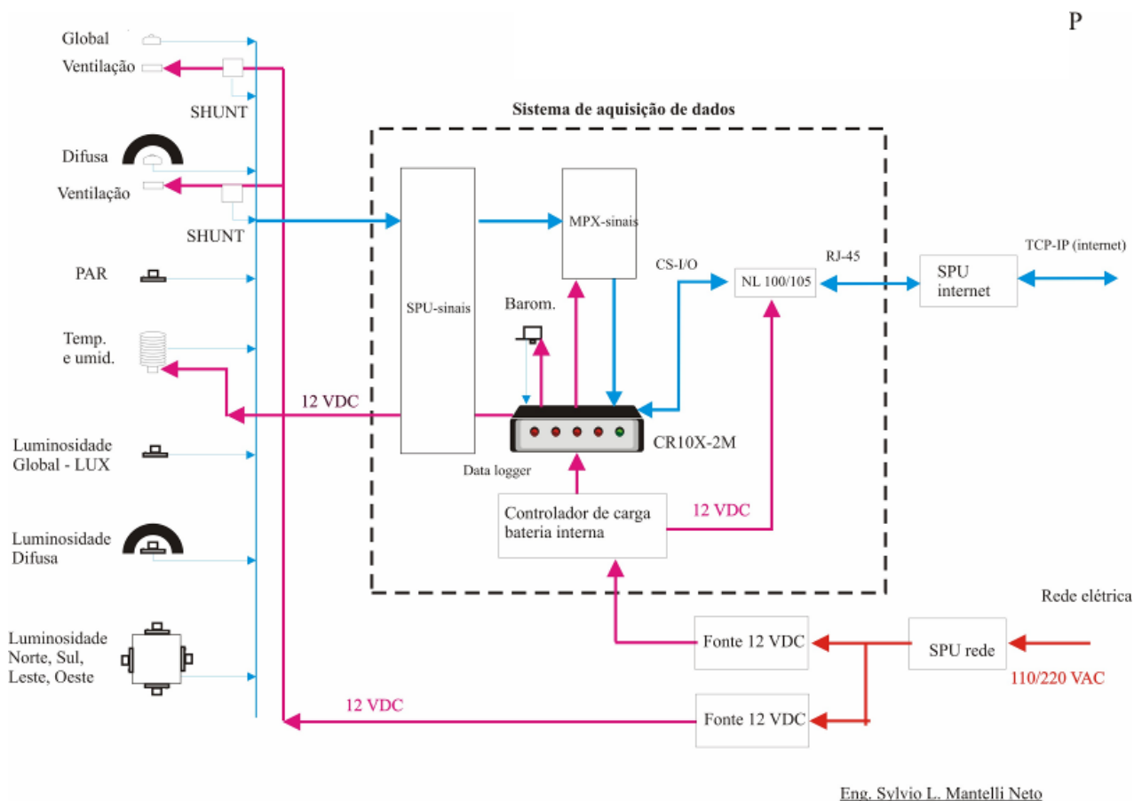
Fig. 6 – Projeto da cadeia de medição da estação solarimétrica e de índice de luminosidade.
