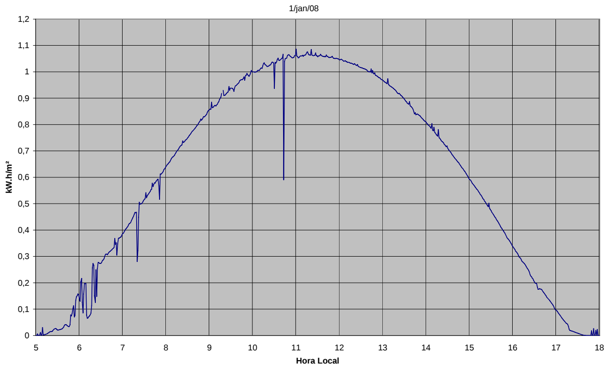
Fig. 16 – Curva da irradiância solar global máxima em 1º de janeiro de 2008.
