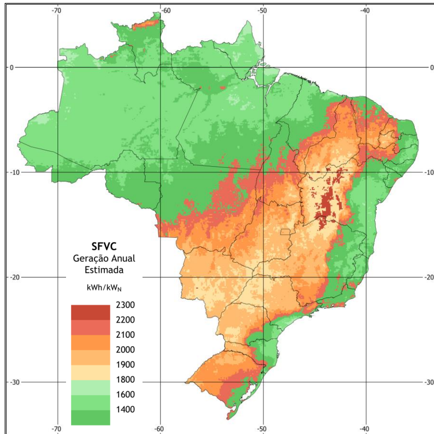
Figura 8 - Mapa de geração fotovoltaica anual estimada, para SFVC, em \text{kWh/kW}_N/\text{ano} .
