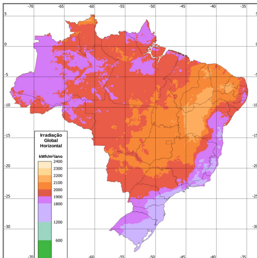
Figura 3 - Mapa do total anual de irradiação global horizontal ( H_{HOR} ), em kWh/m 2 /ano.
