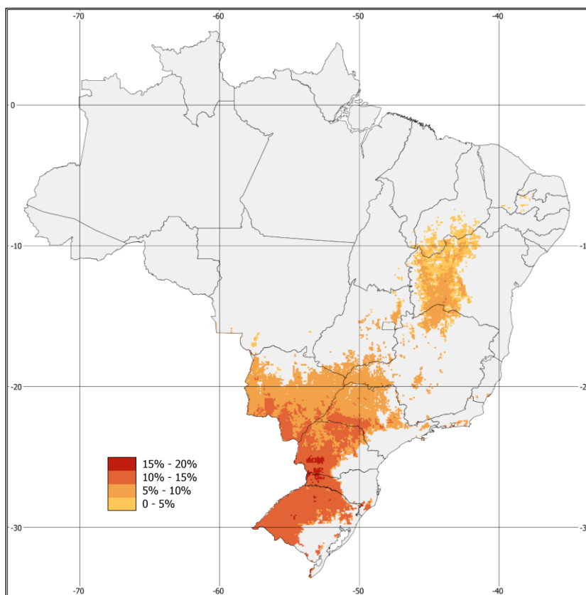
Figura 7 – Mapa que evidencia as áreas nas quais a irradiação direta normal ( H_{DIRN} ) é igual ou maior do que a total ( H_{TOT} ), em %.
