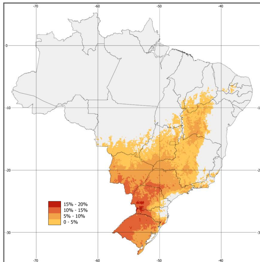
Figura 6 – Mapa que evidencia as áreas nas quais a irradiação direta normal ( H_{DIRN} ) é igual ou maior do que a global horizontal ( H_{HOR} ), em %.
