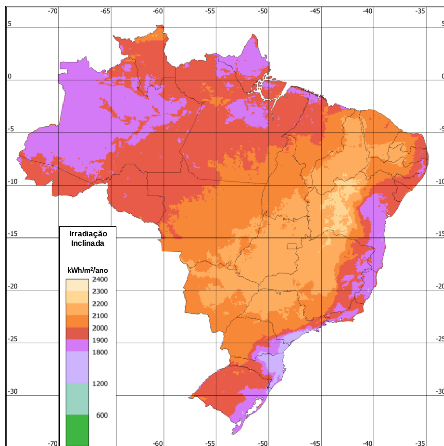
Figura 4 - Mapa do total anual de irradiação total ( H_{TOT} ), em kWh/m 2 /ano, incidente em uma superfície inclinada com inclinação igual à latitude local.
