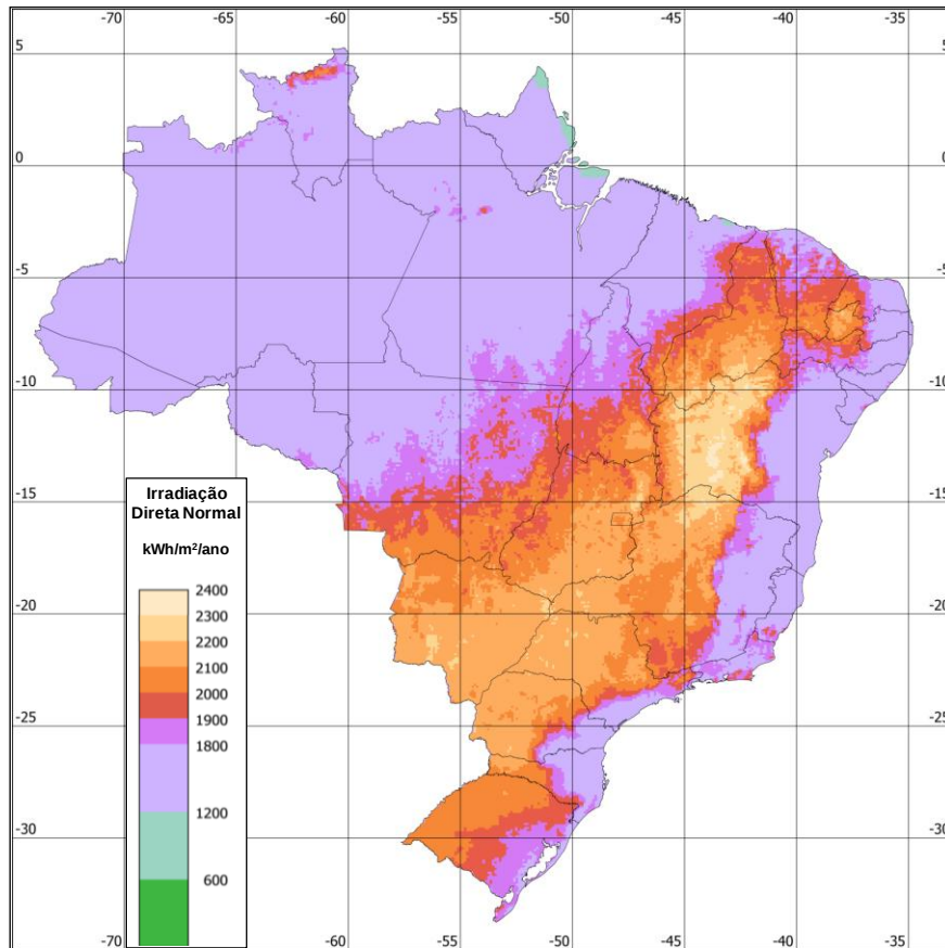
Figura 2 - Mapa do total anual de irradiação direta normal ( H_{\text{DIRN}} ), em \text{kWh/m}^2/\text{ano} .
