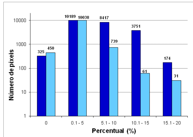
Figura 5 - Histograma com a distribuição de píxeis (área de 10 km x 10 km) para os quais a irradiação direta normal ( H_{DIRN} ) é igual ou maior do que global horizontal (barras escuras, à esquerda) e total (barras claras, à direita).
