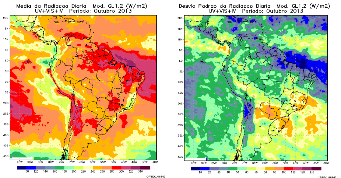
Figura 2 - Média mensal e desvio padrão de irradiância média diária na América do Sul. Unidades: \text{W} \cdot \text{m}^{-2} ( 1 \text{ W} \cdot \text{m}^{-2} acumulado em um dia representa uma irradiação de 0,024 \text{ kWh} \cdot \text{m}^{-2} ).
