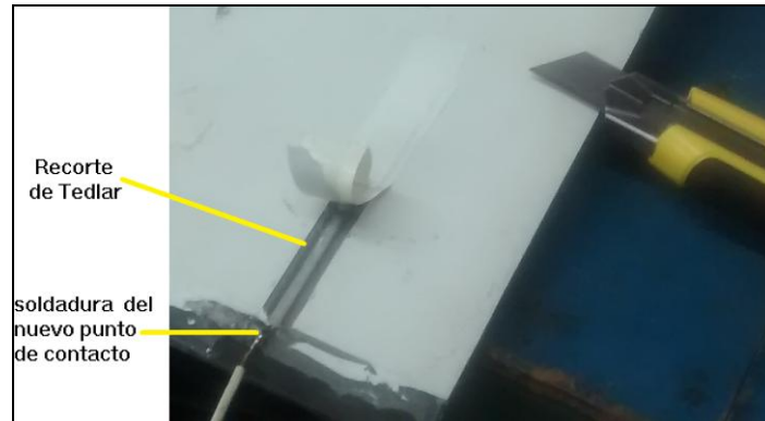
Figura 8 - Cara posterior corte del Tedlar y soldadura
