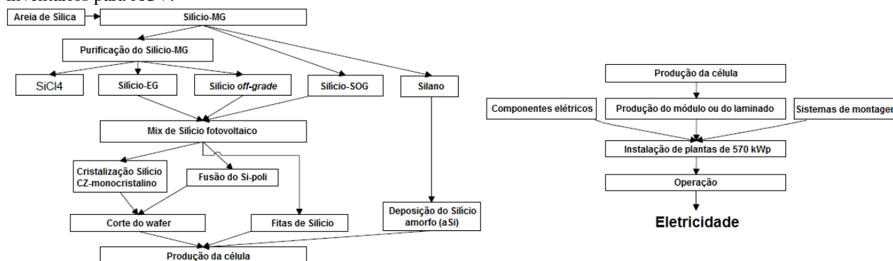
Figura 2 – Processos envolvidos na obtenção de energia solar fotovoltaica. MG-silicon: Silício em grau metalúrgico. EG-silicon: Silício em grau eletrônico. SoG silicon: Silício em grau solar. CZ-sc-silicon: Czochralski silicon crystal. mc-Si: Silício multicristalino. a-Si: Silício amorfo. Fonte: Adaptado de Jungbluth et al. (2010)
