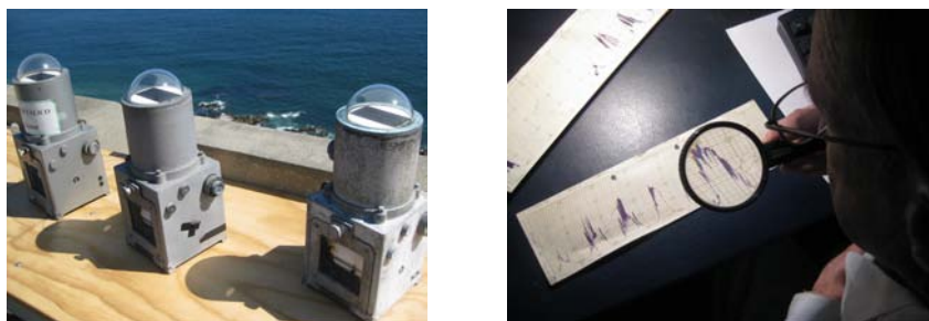
Figura 1 – Actinógrafos del ANS (izquierda) y el Sr. Robero Sotta (dercha) de la UTFSM, revisando mediciones.
