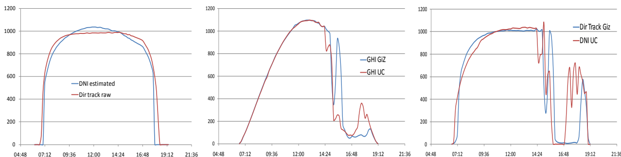
Figura 6 – Comparación de datos en W/m^2 ; CNE-GiZ crudos y reprocesados, para el día 21/09/2010 (izquierda); CNE-GiZ y PUC-FONDEF en San Pedro de Atacama, para el día 01/03/2011 (centro y derecha).
