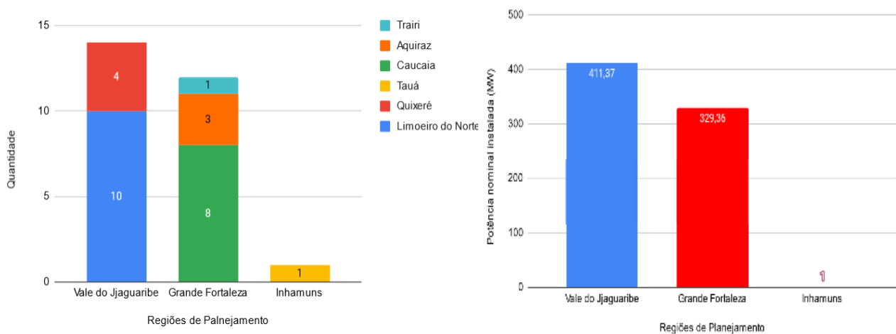
Figura 7 – Distribuição de empreendimentos FVs em operação, por região e por município (a) e potências nominais dos empreendimentos nessas regiões (b).
