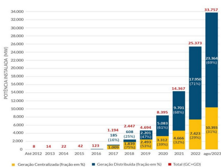
Figura 3 – Evolução da energia solar FV no Brasil. Fonte: ABSOLAR (2023).
