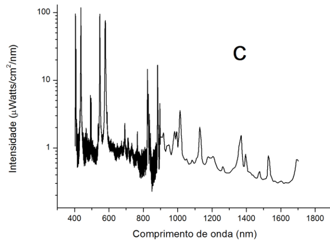
Figura 2 – Irradiância das lâmpadas QTH e de Xe.
