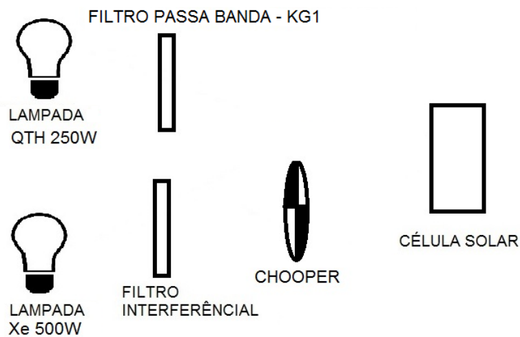
Figura 9 – Configuração para caracterização da junção da base.
