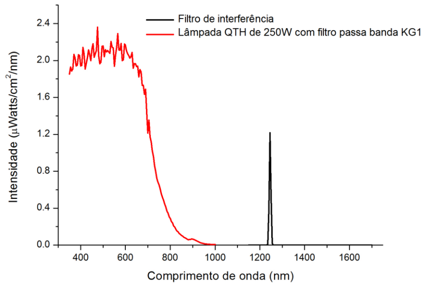
Figura 10 – Espectro para caracterização espectral da junção de base: em vermelho é apresentado o espectro da lâmpada QTH 250W com um filtro passa banda KG1; em preto um filtro interferência de 1250nm como exemplo para a luz de medida.
