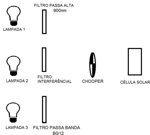
Figura 7 – Configuração para caracterização da junção do meio.
