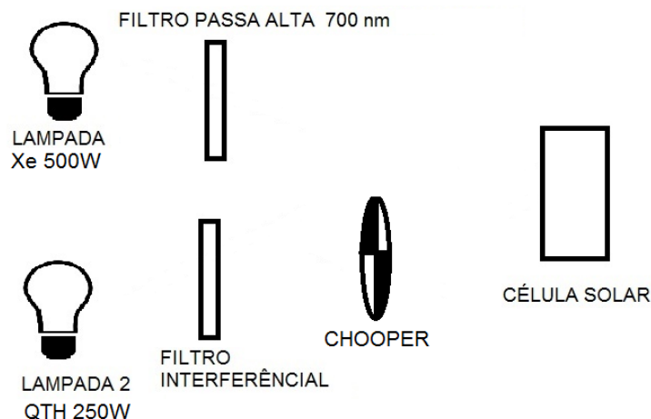
Figura 5 – Configuração para caracterização da junção de topo.
