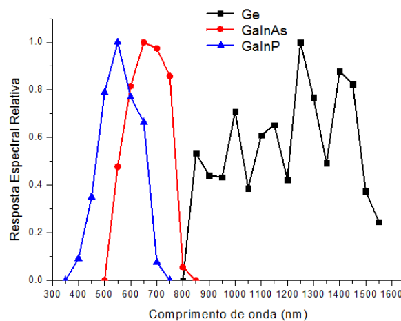
Figura 11 – Resposta espectral de uma célula solar de tripla junção de (GaInP/GaInAs/Ge) do tipo utilizado no satélite CBERS-4.
