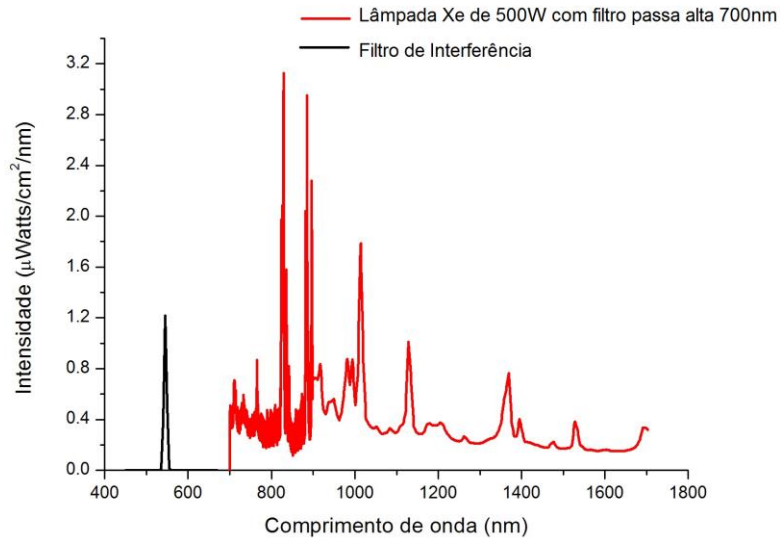
Figura 6 – Irradiância para caracterizar a junção de topo
