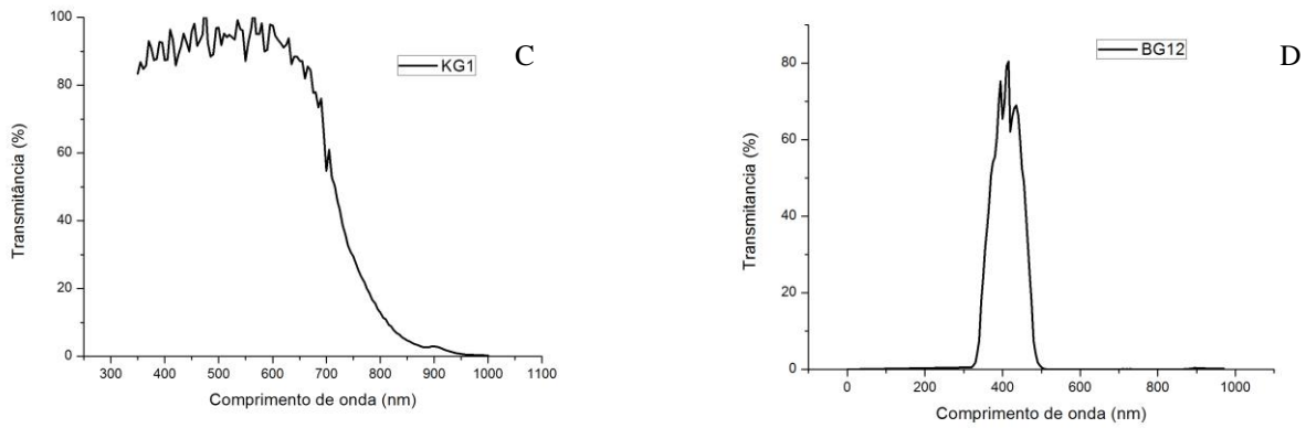
Figura 4 – Transmitância do filtro.
