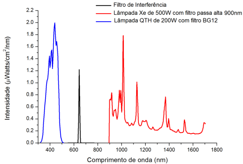
Figura 8 – Espectro para caracterização espectral da junção do meio.
