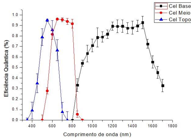
Figura 12 – Eficiência Quântica normalizada da célula solar de tripla junção (GaInP/GaInAs/Ge), conforme obtida das medidas realizadas com o sistema proposto.
