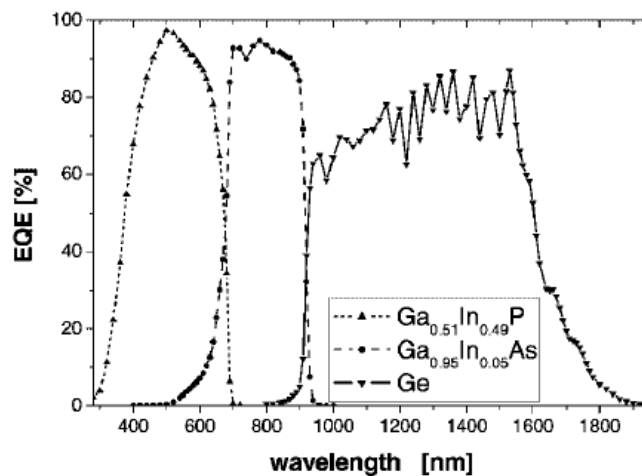
Figura 13 – Resultado obtido da Literatura (Prog. Photovolt: Res. Appl. 2003; 11:499–514 (DOI: 10.1002/pip.514)) Fonte: Meusel (2003).
