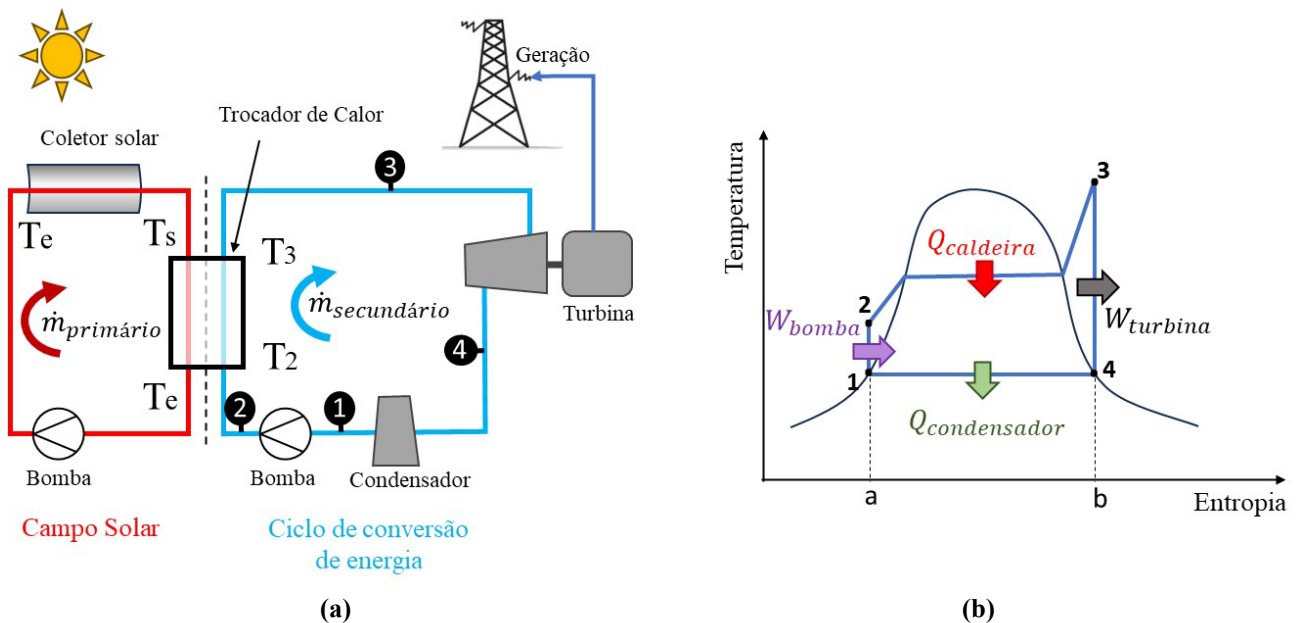
Figura 1 – (a) Representação esquemática de uma usina CSP, (b) Ciclo Rankine simples.
