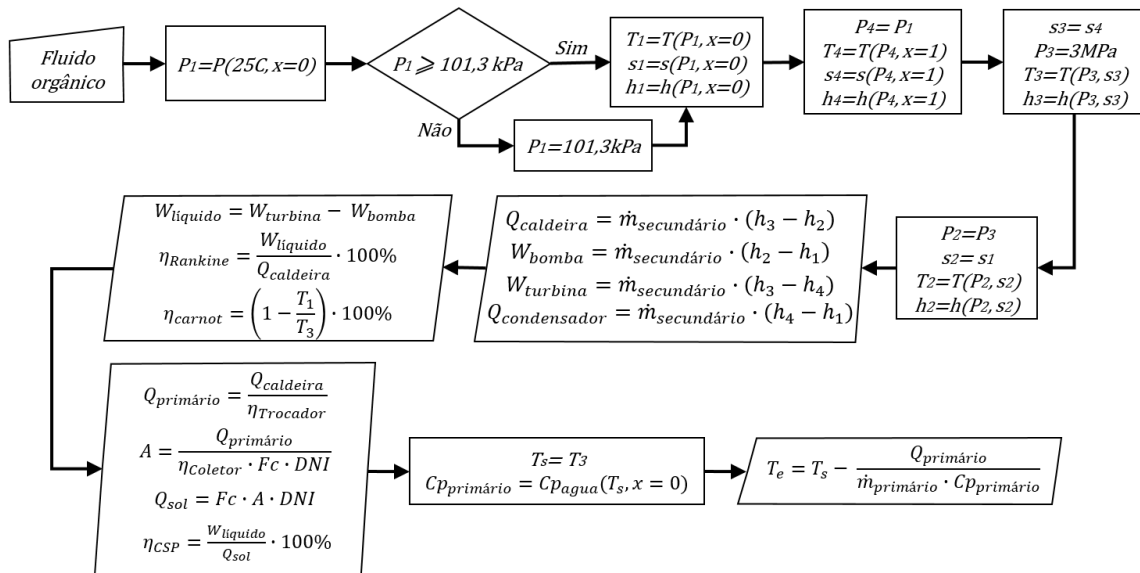
Figura 3 – Fluxograma de cálculo para a usina CSP operando com fluidos orgânicos.
