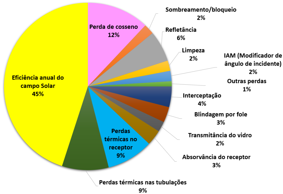
Figura 2 – Eficiência e relação de perdas sofridas por um coletor solar. Fonte: Adaptado de Heller (2017)
