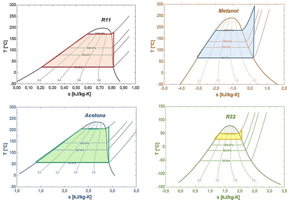
Figura 4 – Ciclo Rankine para alguns fluidos orgânicos analisados.
