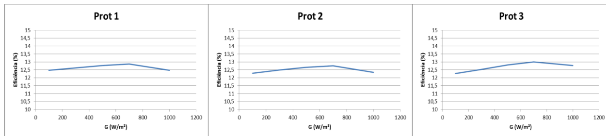
Figura 13 – Variação de eficiência com o aumento da irradiância do Prot 1, Prot 2 e Prot 3 (Fonte: do autor).
