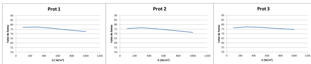
Figura 12 – Variação de FF com o aumento da irradiância do Prot 1, Prot 2 e Prot 3 (Fonte: do autor).
