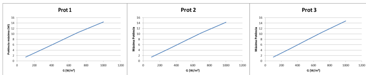
Figura 14 – Variação da P_{MÁX} com o aumento da irradiância do Prot 1, Prot 2 e Prot 3 (Fonte: do autor).
