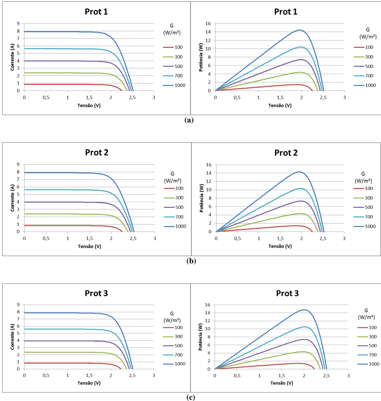
Figura 10 – Curvas I-V e curvas P-V dos Prot 1 (a), Prot 2 (b) e Prot 3 (c) em diferentes níveis de irradiância (Fonte: do autor).
