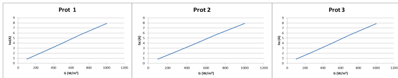
Figura 11 – Relação da I_{SC} com a variação de irradiância do Prot 1, Prot 2 e Prot 3 (Fonte: do autor).
