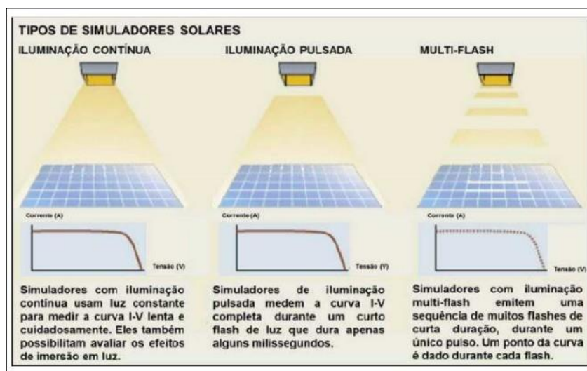
Figura 8 – Exemplos de simuladores solares (Dalmagro, Krenzinger, 2013).
