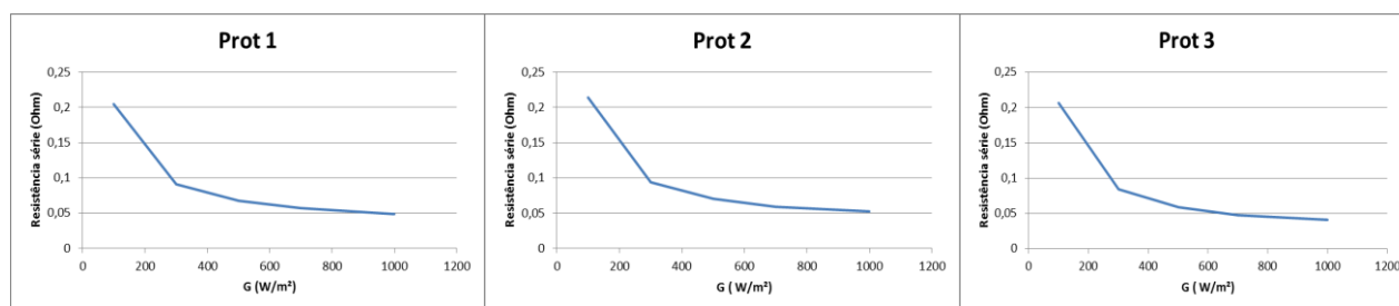
Figura 15 – Variação da R_S com o aumento da irradiância do Prot 1, Prot 2 e Prot 3 (Fonte: do autor).
