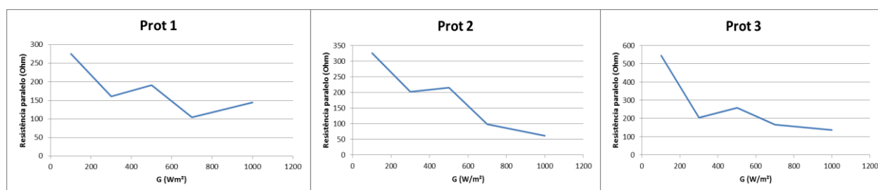
Figura 16 – Variação da R_P com o aumento da irradiância do Prot 1, Prot 2 e Prot 3 (Fonte: do autor).
