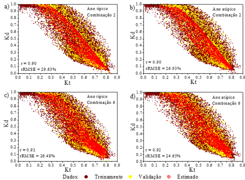
Figura 4: Dispersão da estimativa de k_d calculada pela rede neural do tipo RBF em função de k_t .
