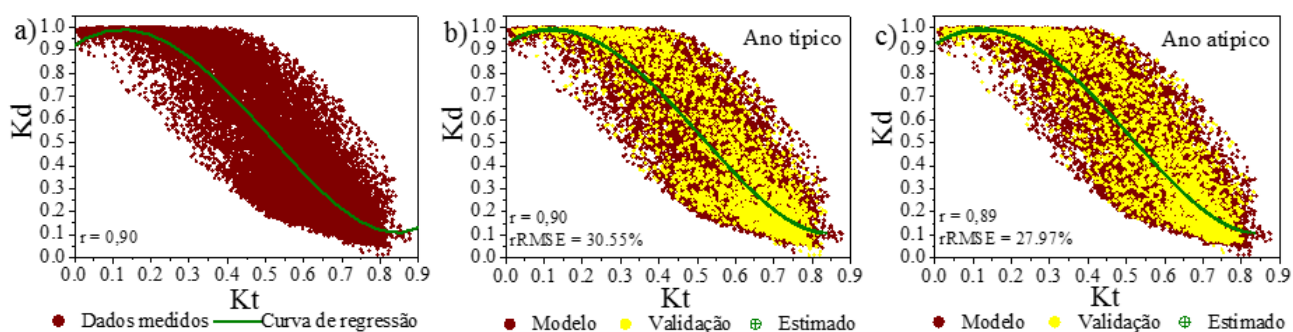
Figura 3: a) Curva de dispersão de k_t em relação a k_d com todos os dados; curva de dispersão de k_d com dados de validação e valor estimado para: b) Ano típico (AT); c) Ano atípico.
