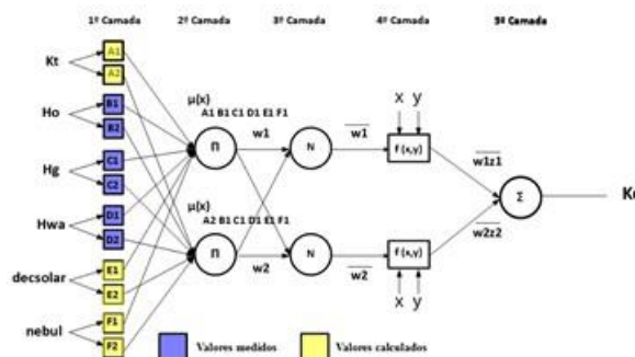
Figura 2: Arquitetura da ANFIS. Adaptado de Jang, 1993.
