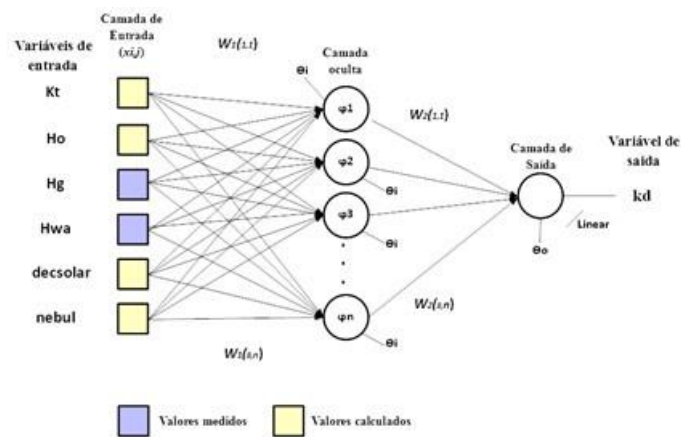
Figura 1: Arquitetura da Rede Neural de Base Radial. Adaptado de Silva et al, 2010.
