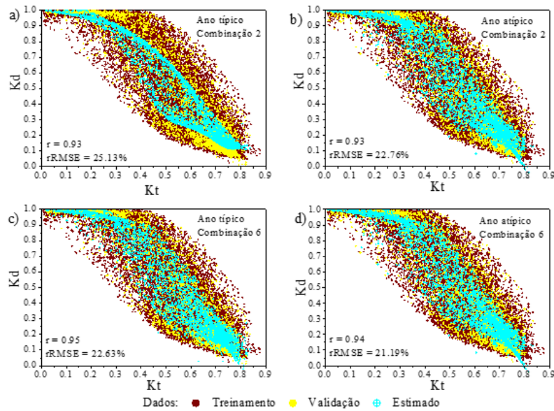
Figura 5: Dispersão da estimativa de k_d calculada pela rede neural do tipo ANFIS em função de k_t .
