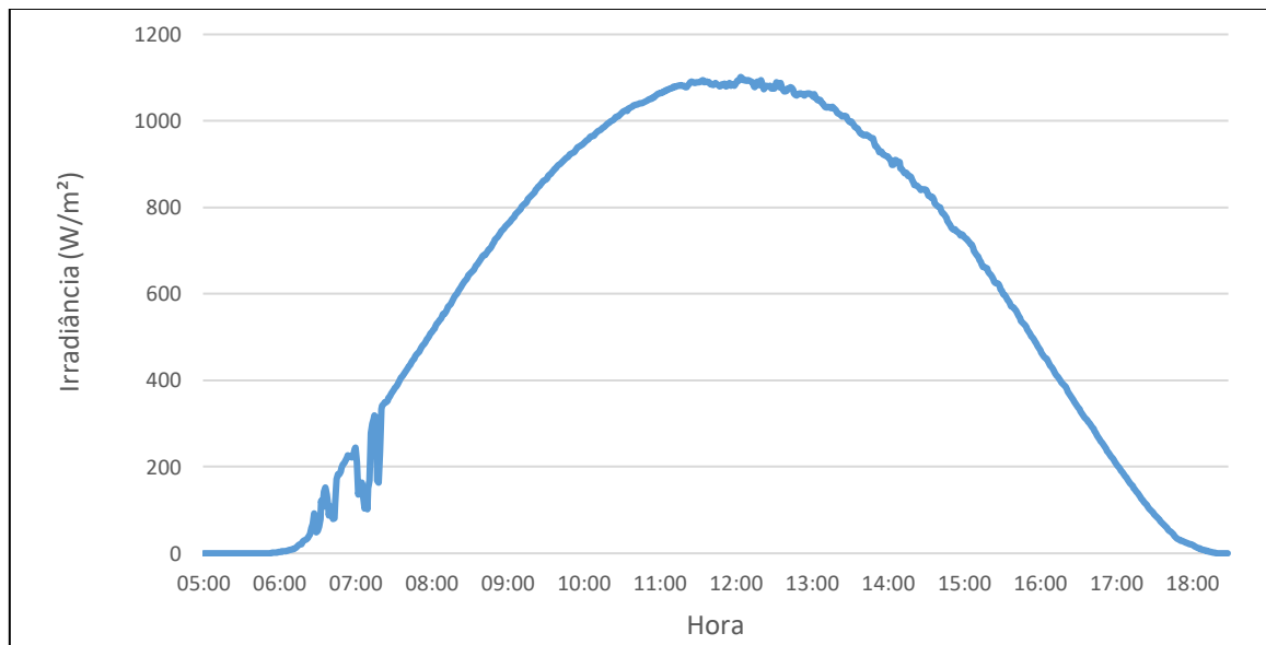
Figura 2 – Irradiância global no plano inclinado na latitude no dia 01/10 de 2019.
