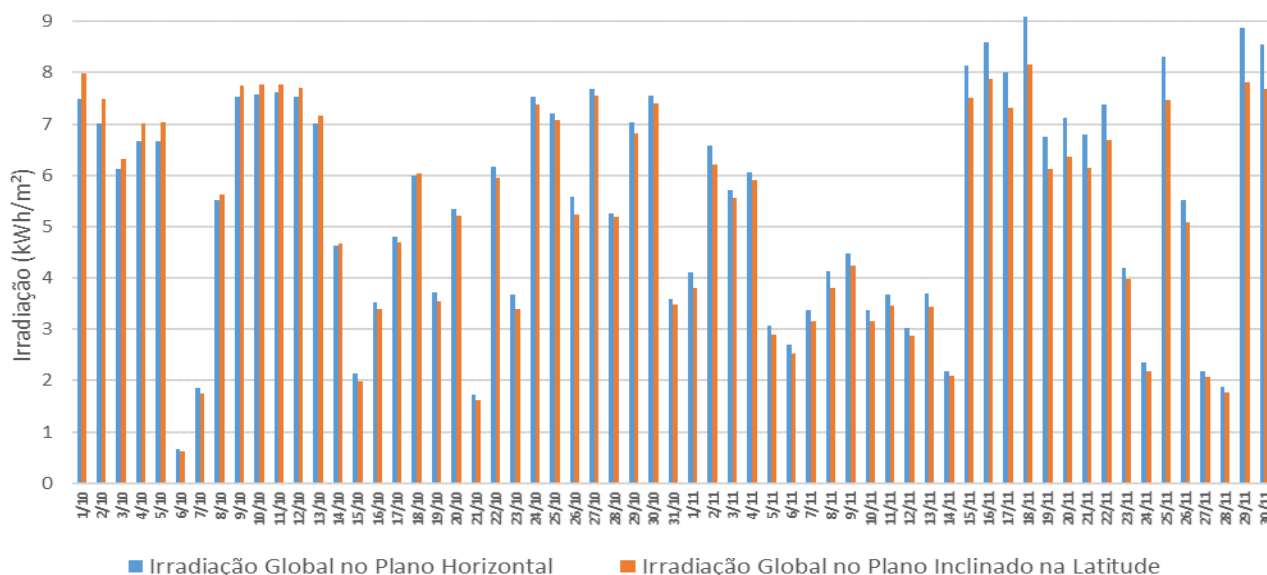
Figura 5 – Irradiação global diária no plano horizontal e inclinado na latitude.
