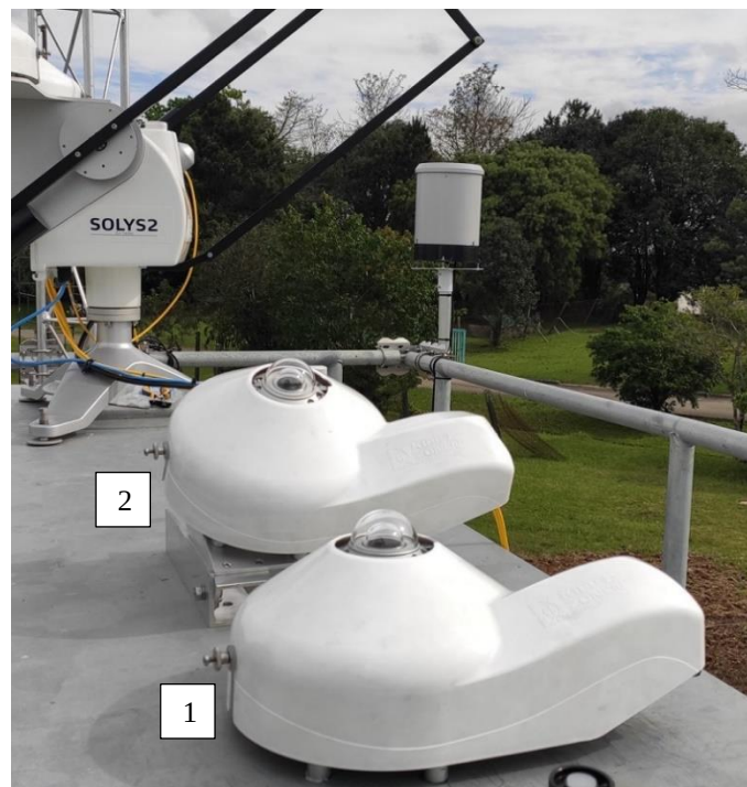
Figura 1 – Piranômetros no plano horizontal (1) e inclinado (2).
