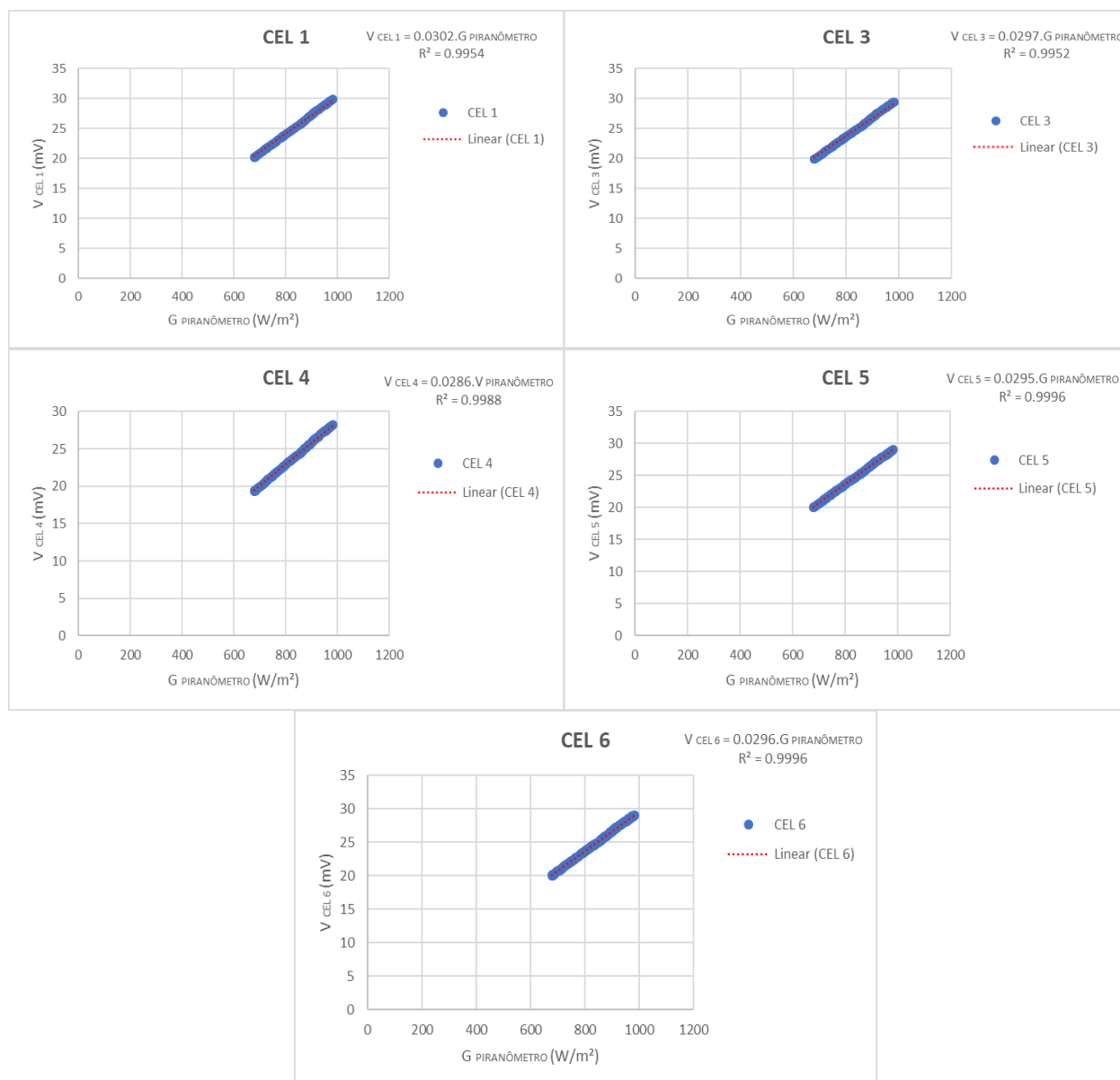
Figura 11 - Curva de calibração ( outdoor ) para as células de referência utilizando o piranômetro térmico padrão (calibrado).
