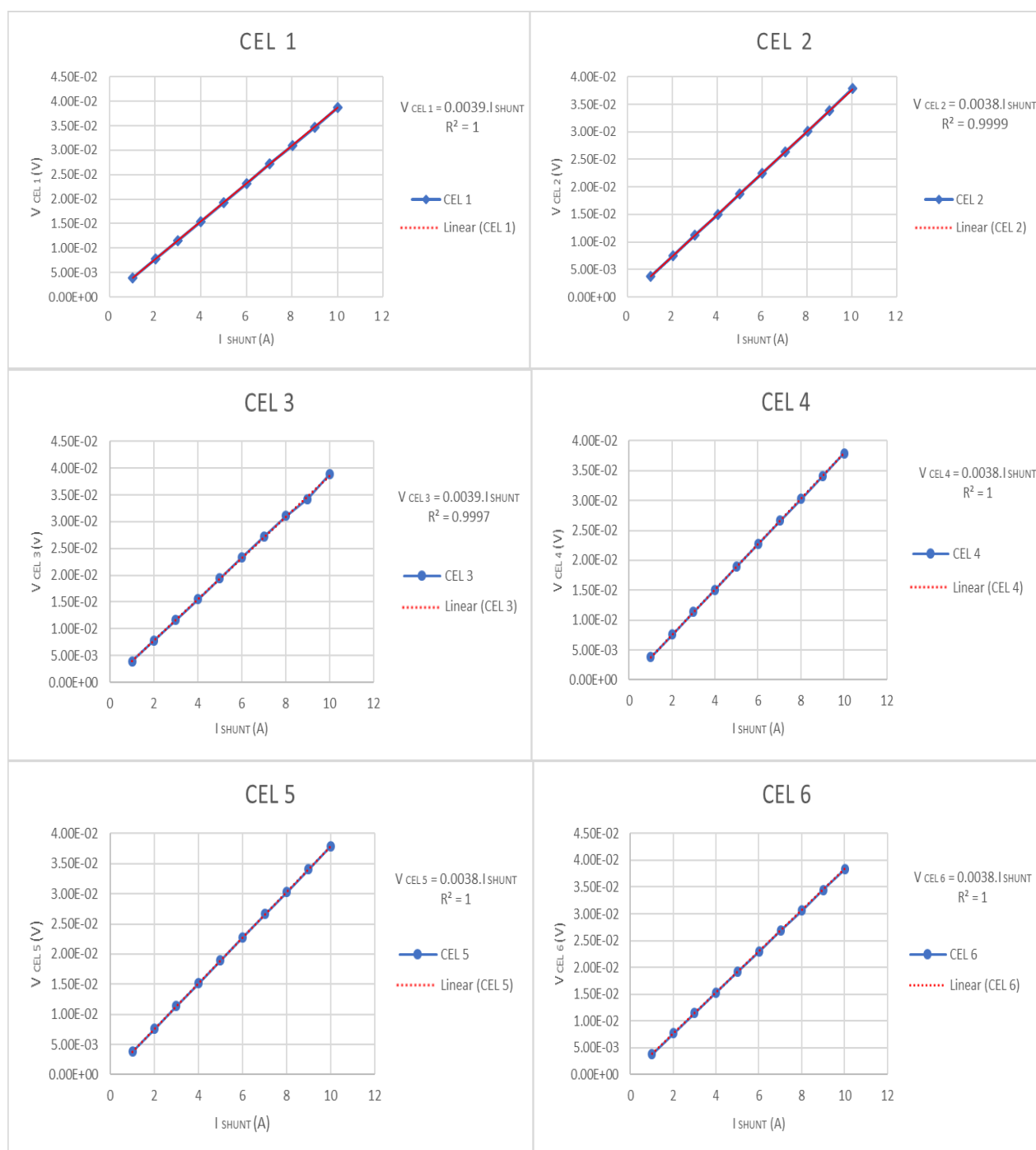
Figura 12 - Curva de calibração ( outdoor ) para as células de referência utilizando o piranômetro térmico padrão (calibrado).
