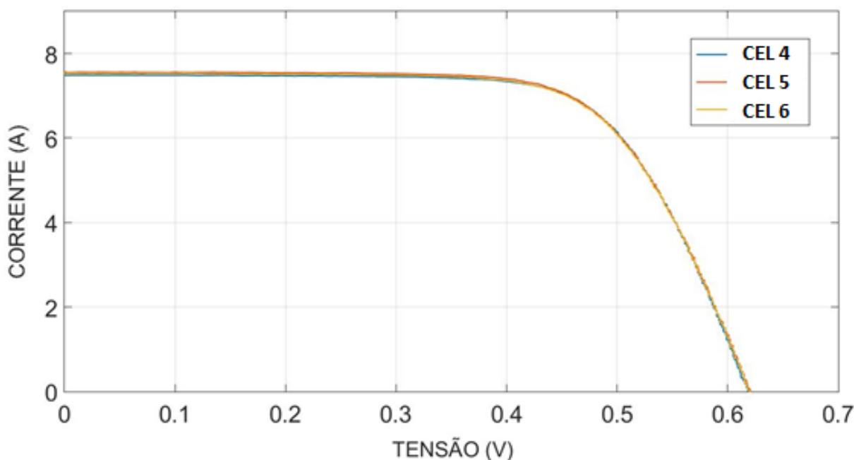
Figura 9 – Curvas I-V das células de referência de mc-Si, G = 1000 \text{ W/m}^2 , T_{\text{célula}} = 25 \text{ }^\circ\text{C} e AM1,5.
