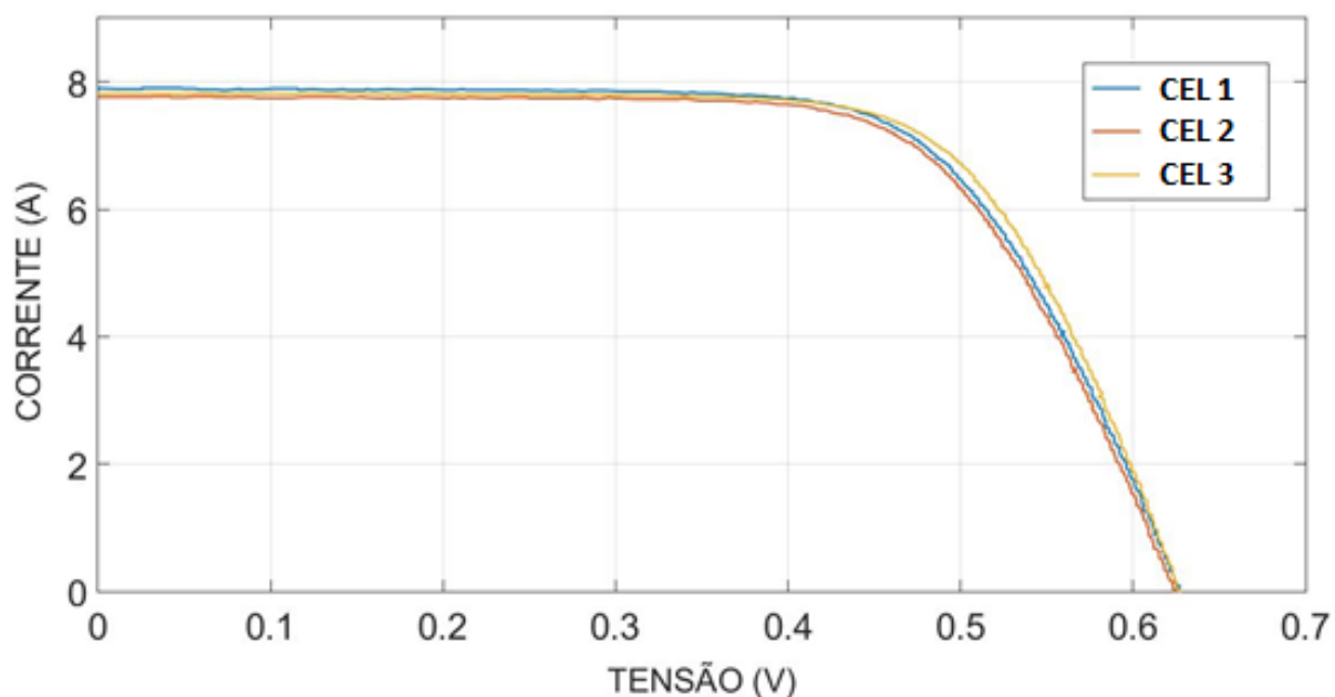
Figura 8 – Curvas I-V das células de referência de m-Si, G = 1000 \text{ W/m}^2 , T_{\text{célula}} = 25 \text{ }^\circ\text{C} e AM1,5.
