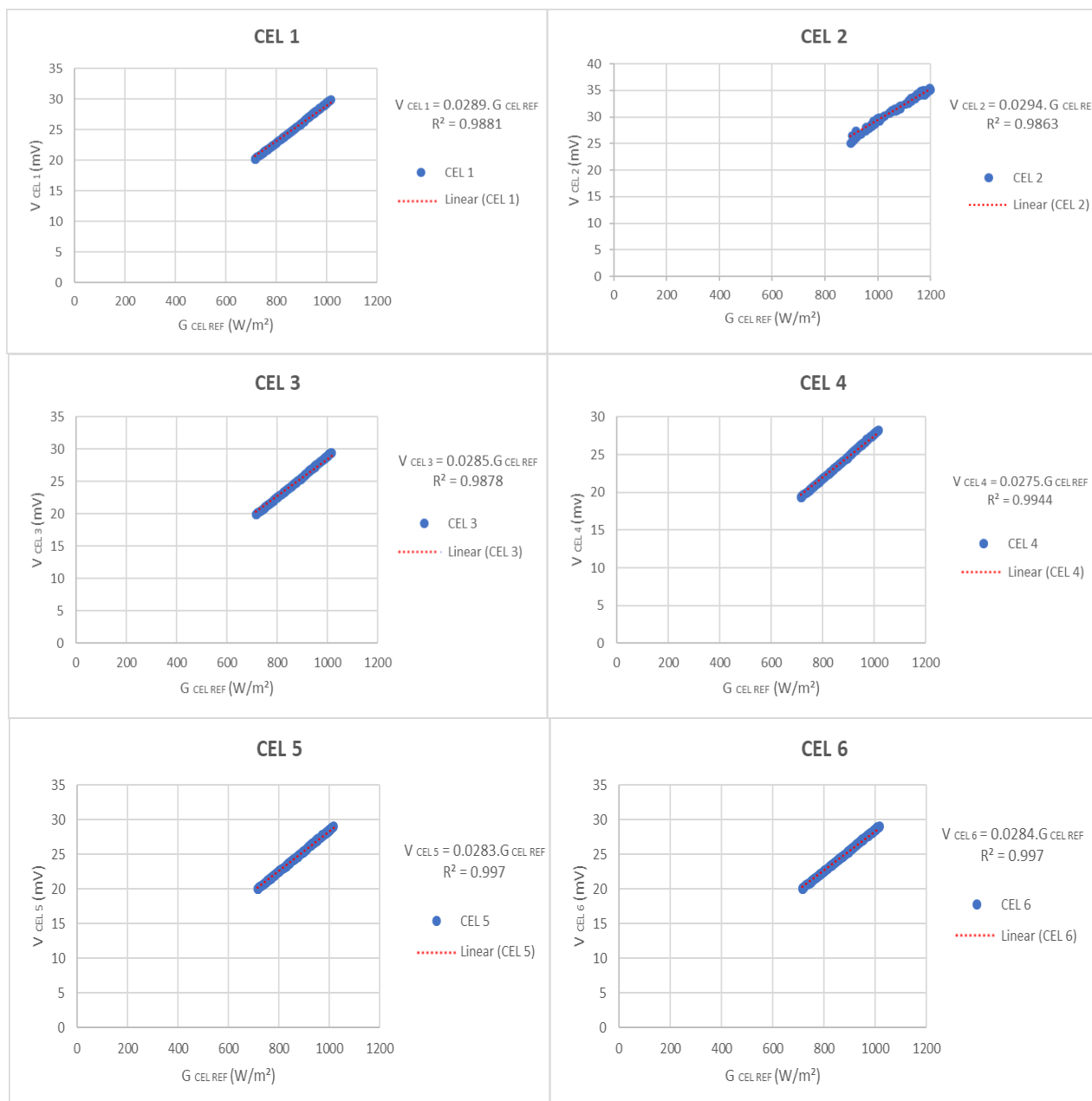
Figura 10 - Curva de calibração ( outdoor ) para as células de referência utilizando a célula de referência padrão (calibrada).
