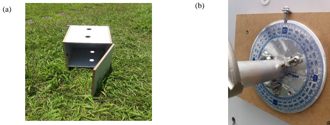
Figura 3 – (a) Dispositivo parcialmente montado. (b) Eixo com disco graduado para alteração do ângulo do piranômetro
