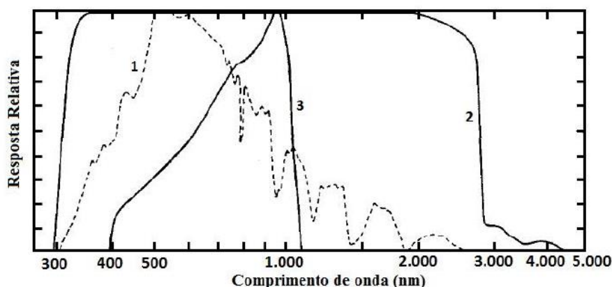
Figura 2 – Comparativo entre respostas espectrais dos diferentes tipos de piranômetros. 1 – Distribuição espectral da irradiância solar na superfície da Terra. 2 – Resposta do piranômetro termoelétrico. 3 – Resposta do piranômetro FV (silício). Fonte:(Alados-Arboleta et al., 1995 apud Pinho J.T. et al., 2014)
