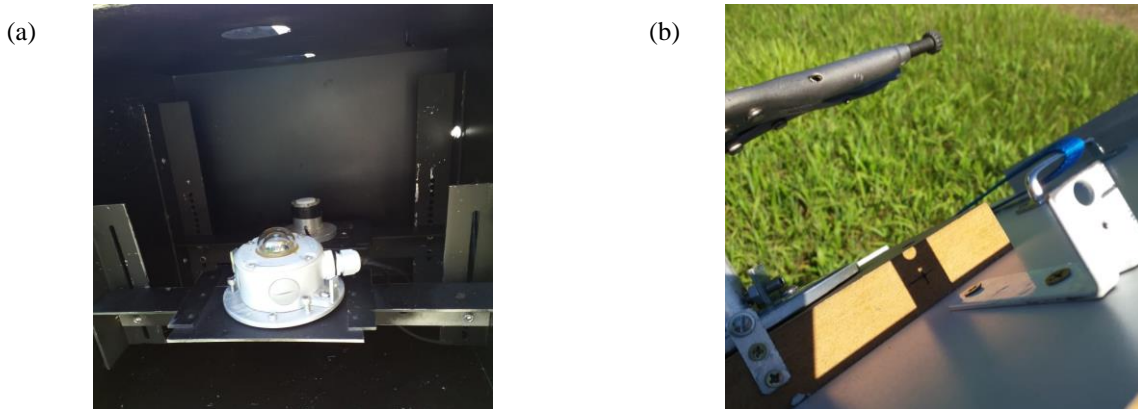
Figura 4 – (a) Suportes internos para os piranômetros. Ao fundo está um piranômetro fotovoltaico com função de verificação da estabilidade da radiação durante ensaio de resposta angular. No primeiro plano é possível ver o protótipo montado no suporte giratório com ajuste de altura. (b) mira montada no dispositivo
