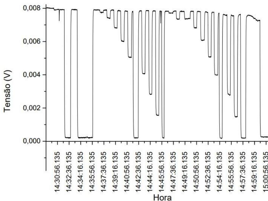
Figura 7 – Gráfico de tensão ao longo do tempo de um piranômetro padrão secundário. Os valores próximos a zero são com a radiação bloqueada. Os valores próximos ao máximo são com radiação direta normal, e os valores intermediários correspondem aos diferentes ângulos de incidência. Na primeira sequência foram medidas as respostas angulares a leste (14h35min até 14h47min) e na segunda sequência as medidas a oeste.
