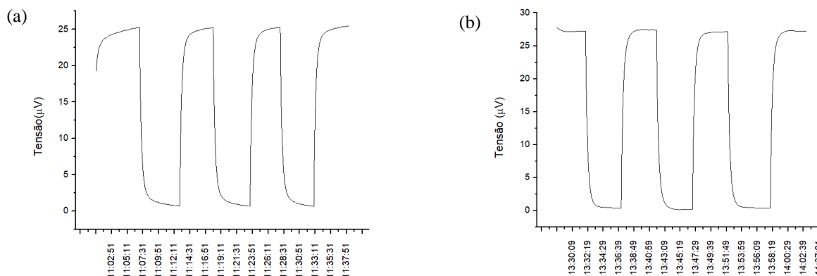
Figura 6 – Gráfico de tensão ao longo do tempo nos ensaios de tempo de resposta do piranômetro protótipo. (a) Das 10h58min até às 11h38min os ensaios foram realizados dentro da caixa colimadora. (b) Das 13h33min até as 14h, os ensaios foram realizados com o piranômetro fora da caixa.
