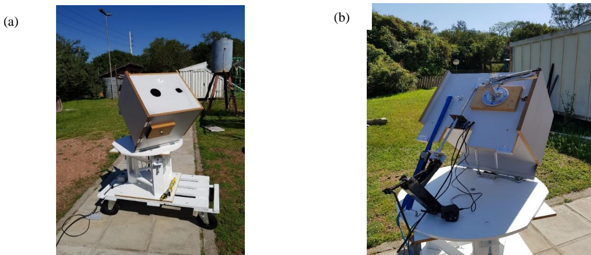
Figura 5 – (a) Dispositivo colimador finalizado e já equipado com o suporte móvel. (b) Visão traseira do dispositivo, com destaque ao macaco, barra roscada e amortecedores, cinta de segurança azul e disco graduado para ajuste de ângulo.
