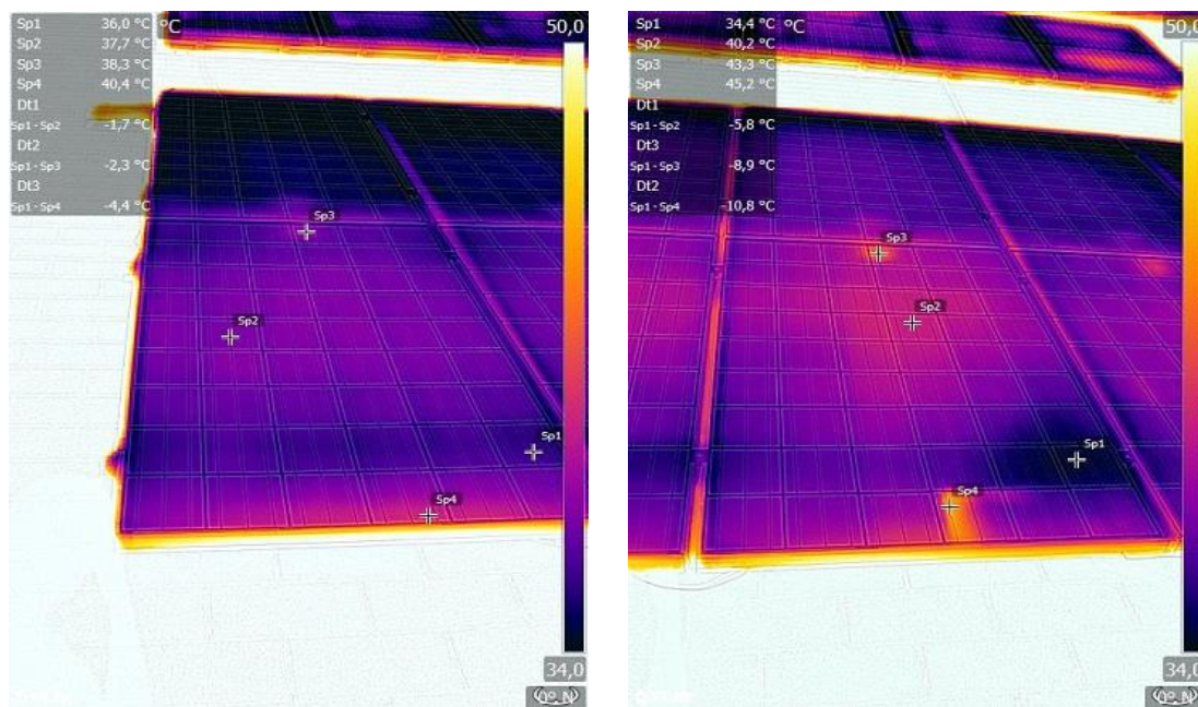
Figura 4(b) - Módulos do EV com pontos quentes.
