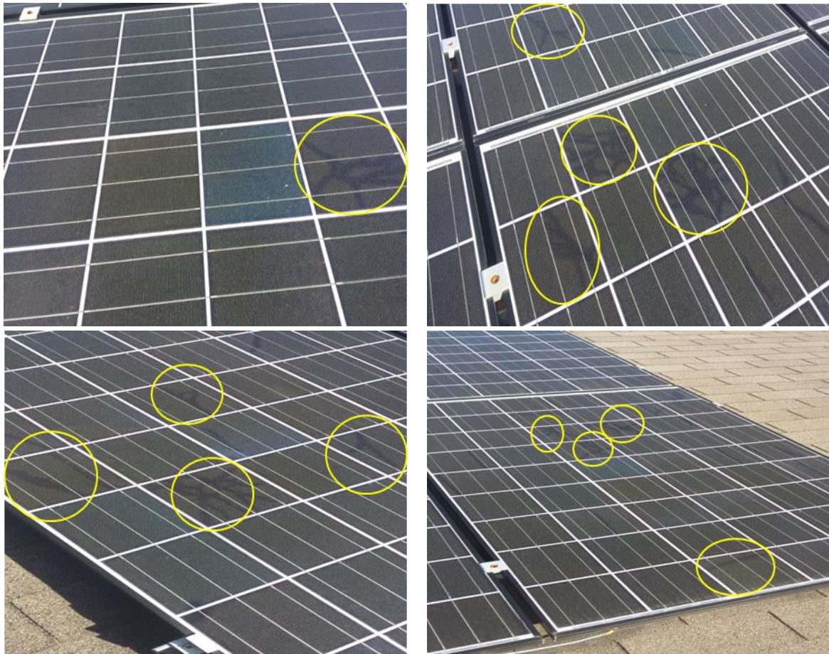
Figura 3 - Módulos do EV com Snail Trail .
