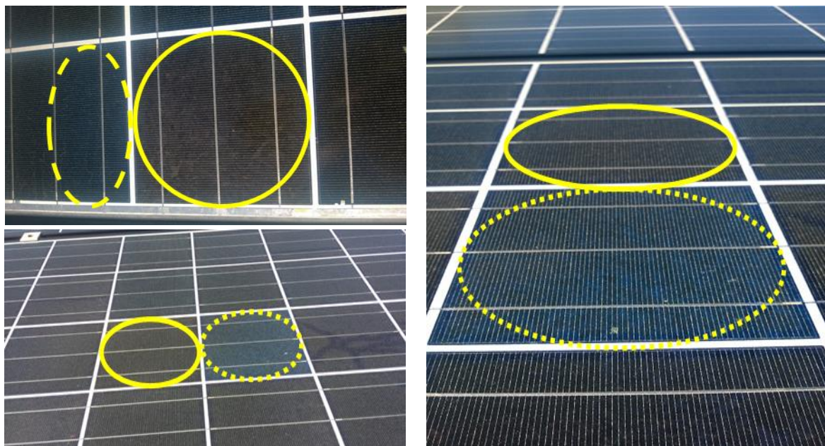
Figura 2 - Módulos do EV com browning .
