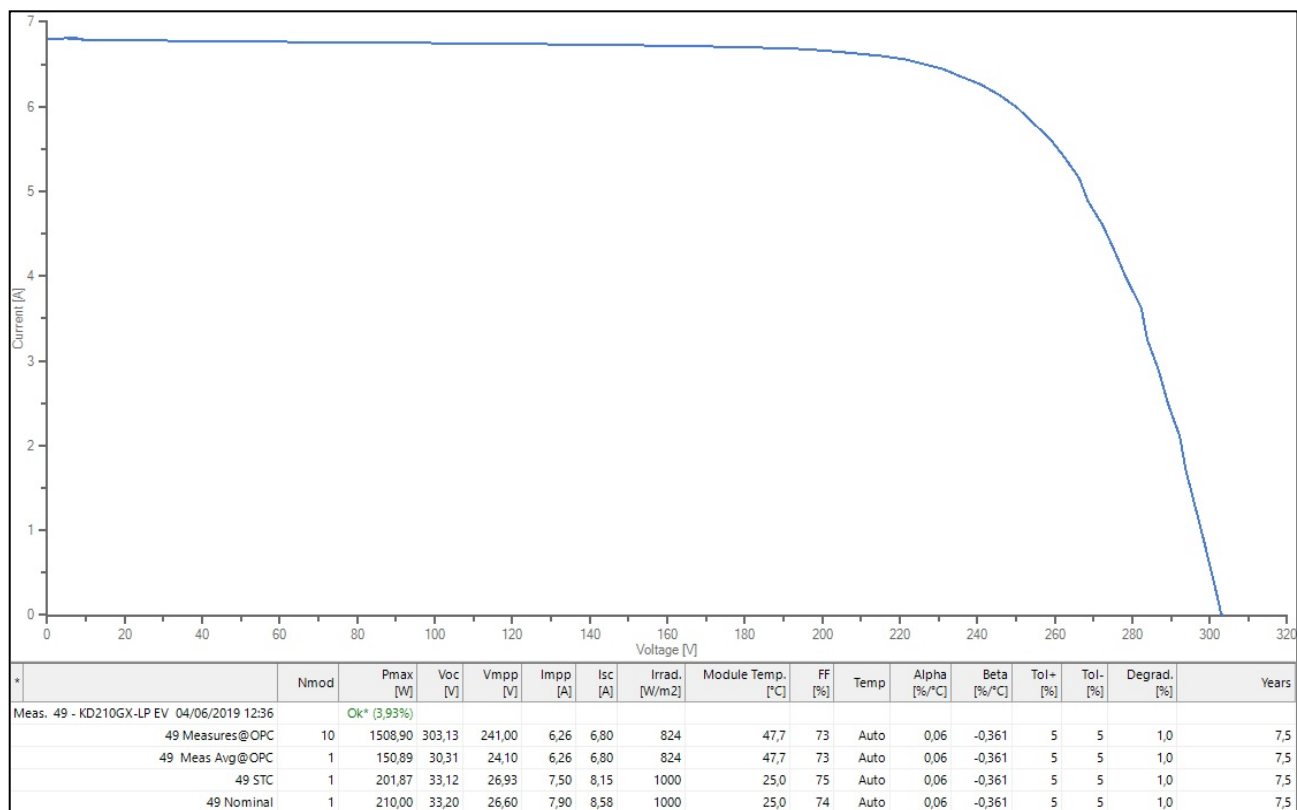
Figura 5 - Gráfico I-V do painel do EV.
