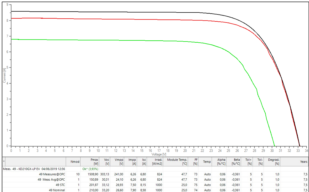
Figura 6 - Gráfico I-V do EV.
