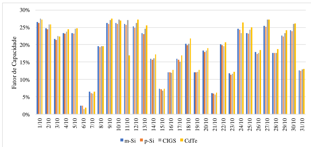
Figura 6 – Fator de capacidade diário das diferentes tecnologias.
