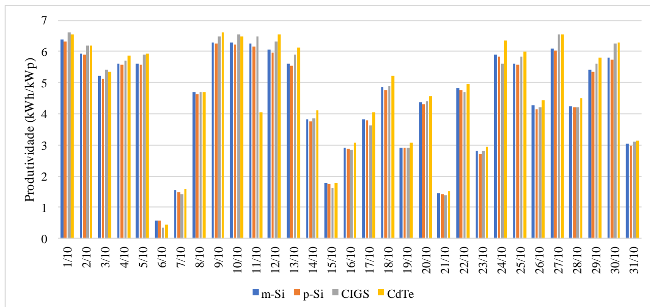
Figura 7 – Produtividade diária das diferentes tecnologias.
