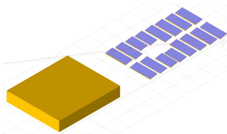
Figura 2 – Modelo tridimensional simplificado do Centro de Eventos e do gerador de 1 MWp no software PVsyst.
