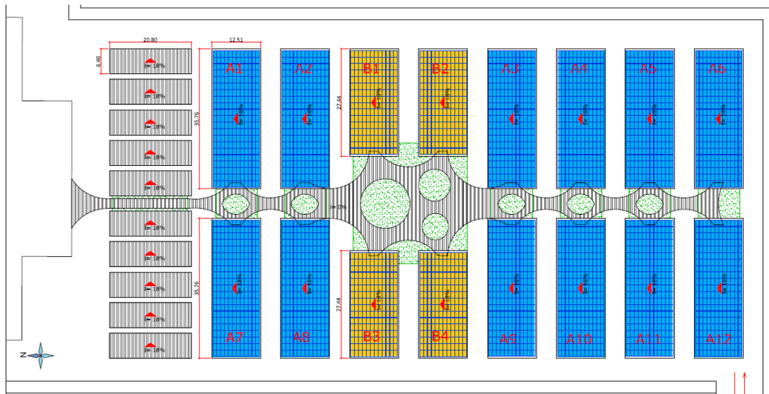
Figura 7 - Divisão de subsistemas do gerador de 1 MWp.
