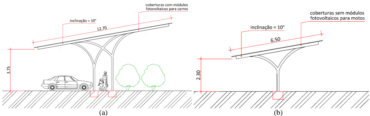
Figura 8 - Desenho dos pilares em “Y curvo” para suporte das coberturas do estacionamento de 1 MWp, sendo (a) para carros e (b) para motos.
